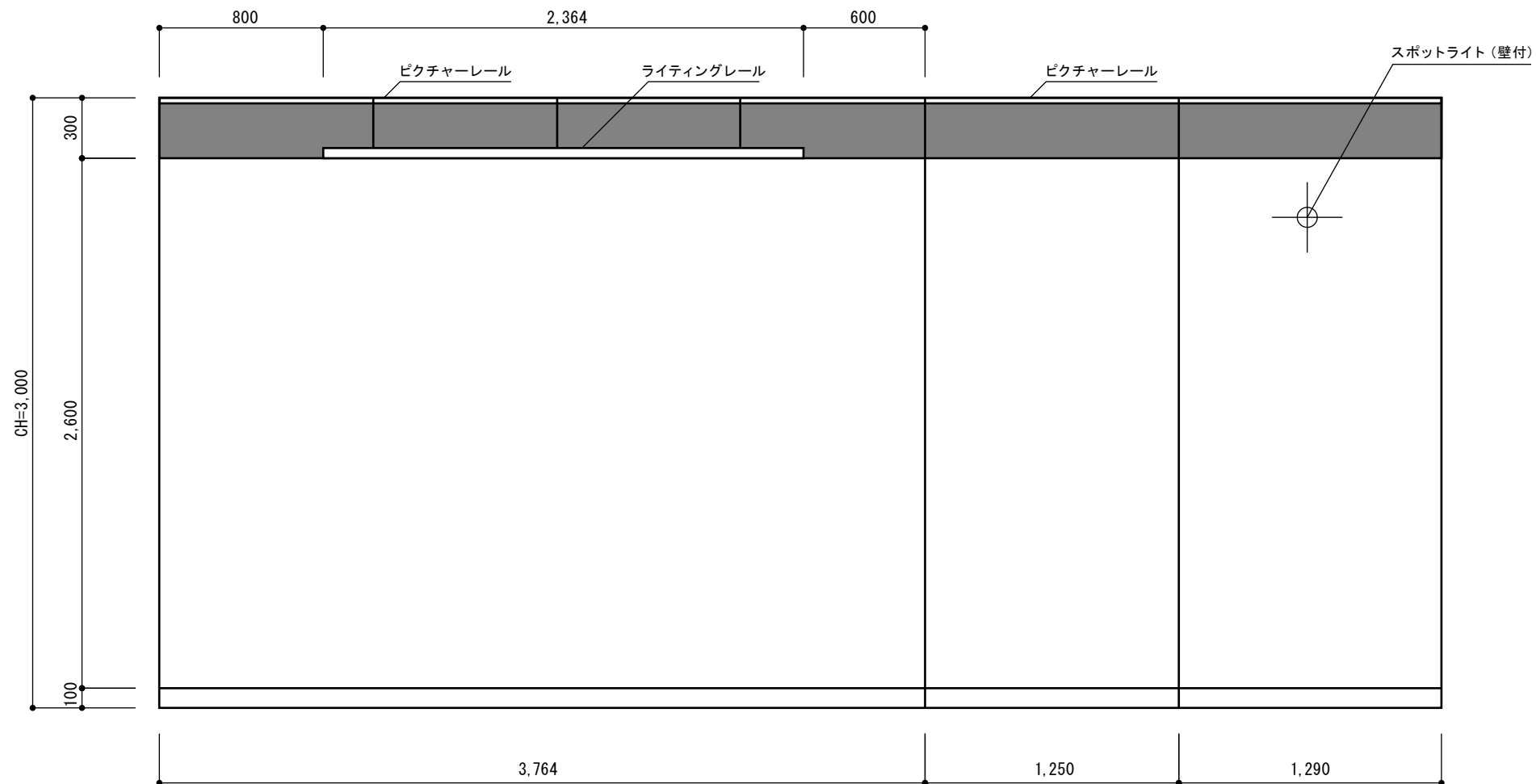
展開図 - C
