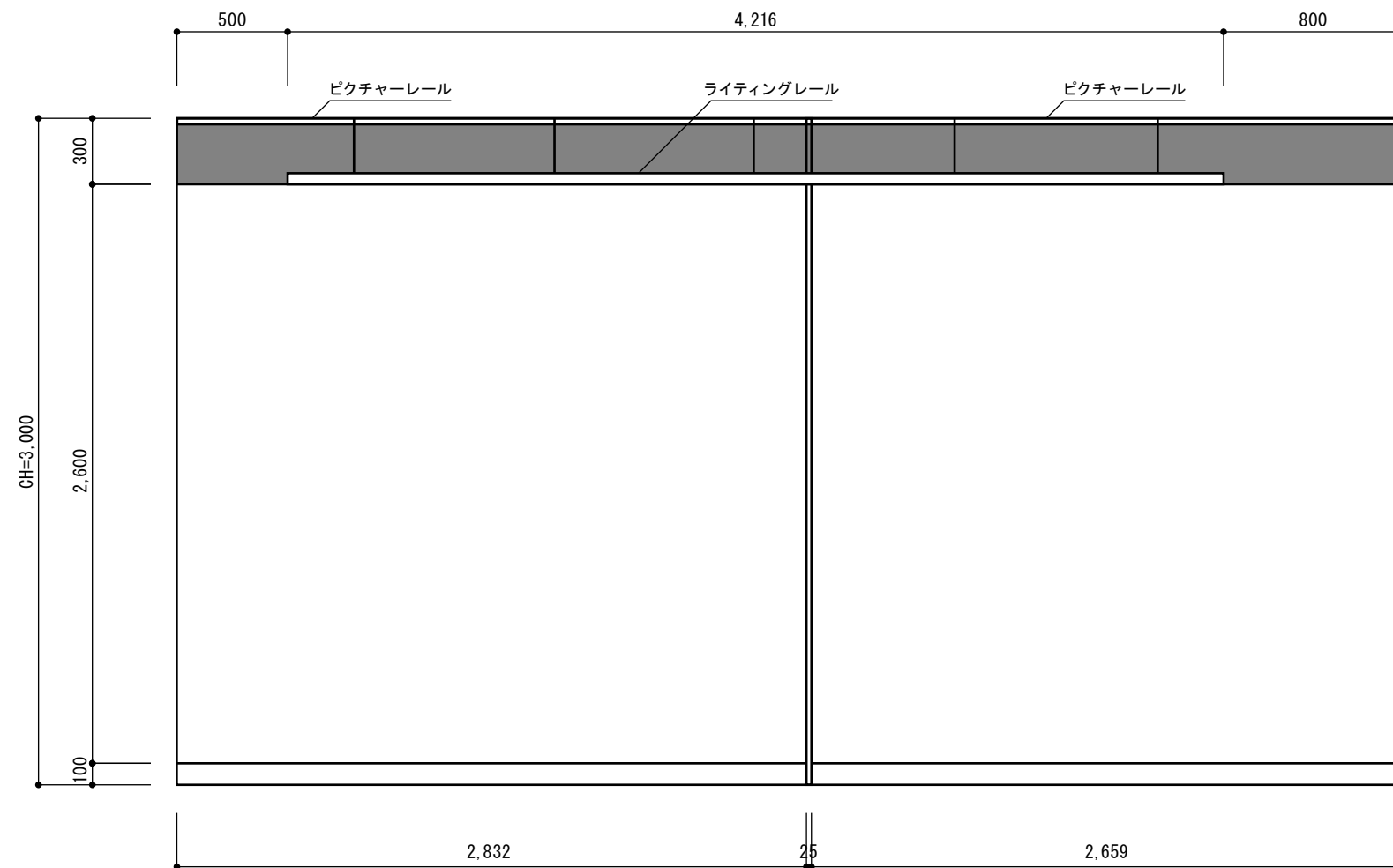
展開図 - A
